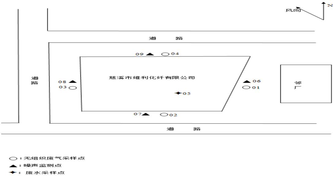
图 3-2 无组织废气及噪声监测点位分布图
